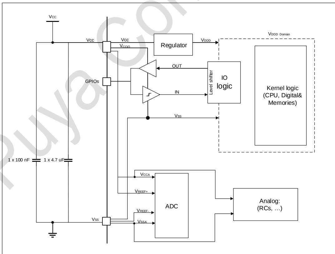
图 5-1 供电方案图
