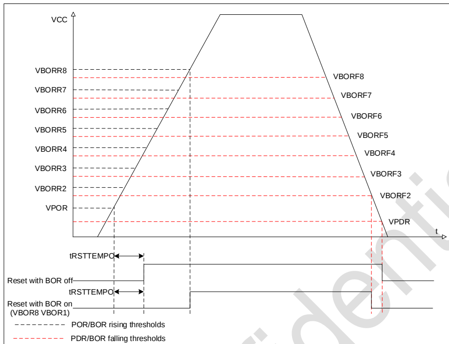
图 2-3 POR/PDR/BOR 阈值
